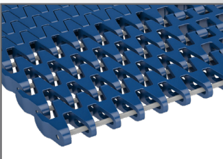
Das aufgewertete Endmodul der Rexnord MatTop-Kette der 1275-1285-Serie
